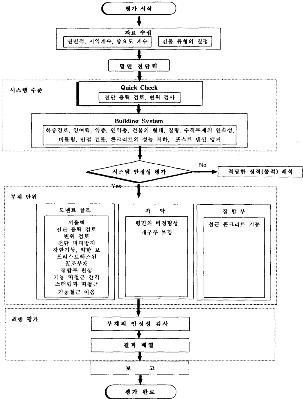
그림 1. 내진 진단의 흐름 (미국)
