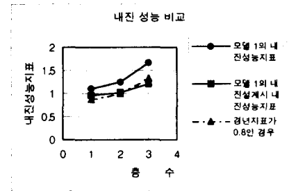
그림 4. Y축 방향에 대한 내진성능평가
