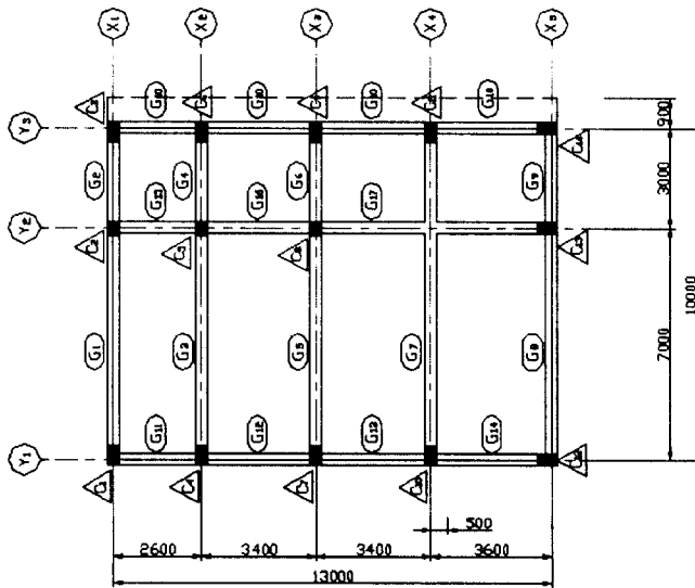
그림 2. 모델 1의 평면도
