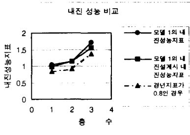
그림 3. X축 방향에 대한 내진성능 평가
