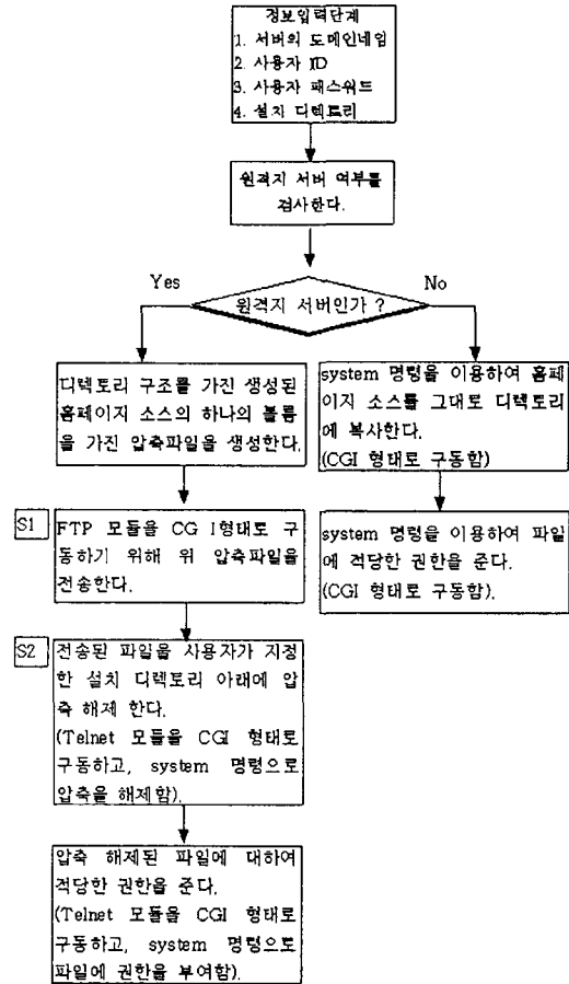
그림 11. 홈페이지 설치자동화 시스템의 수행절차 Fig. 11 Execution procedure of the automation system for homepage installation
