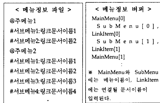
그림 4. 메뉴정보 파일과 버퍼의 구조 Fig. 4 Structure of menu information file and buffer
