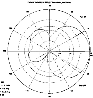
그림 10. E-평면 방사패턴 Fig 10. The radiation pattern of E-plane
