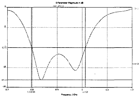
그림 8. 시뮬레이션 반사손실 Fig 8. The simulated return-loss
