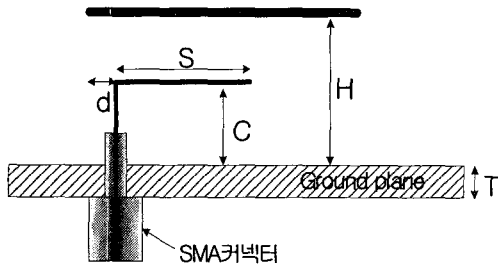
그림 4. 급전 구조 Fig 4. Structure of Feed
