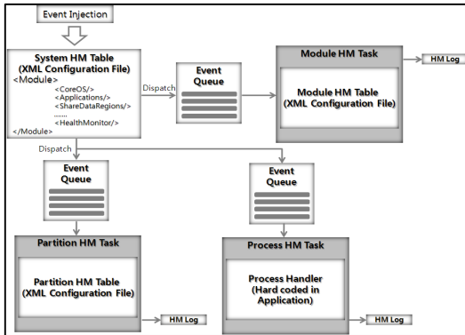
그림 2. HM Architecture
