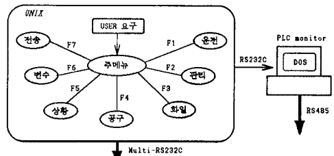
그림 5 운용 시스템 구조
