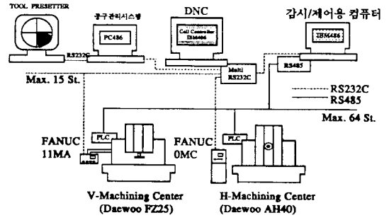
그림 2 하드웨어 구성도
