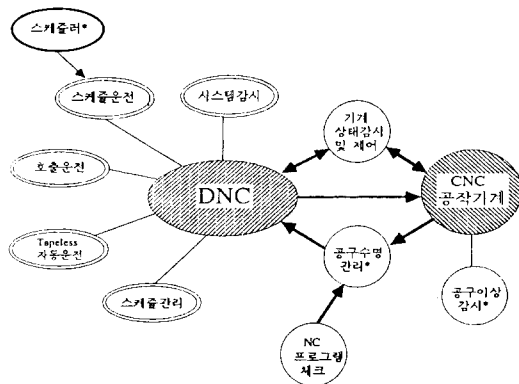
그림 1 DNC 기능구조
