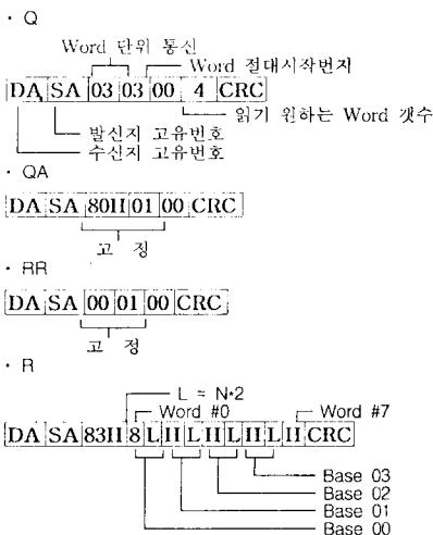
그림 4. RS-485 통신 프로토콜(모니터링 경우)
