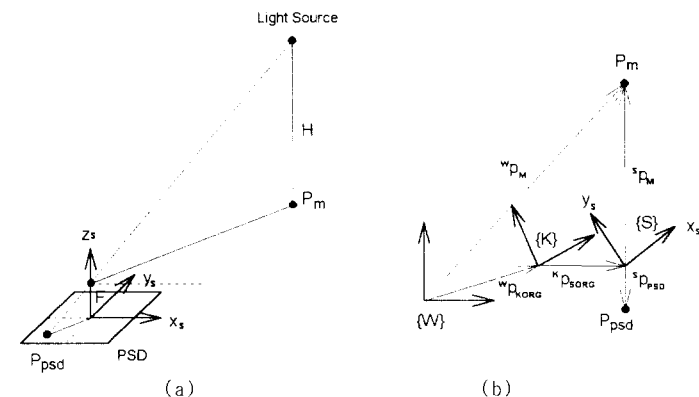
그림 2. (a) 광원과 PSD 좌표계 (b) 주행평면으로의 투영 Fig. 2. (a) Light source and PSD coordinates (b) Projection to navigation planes
