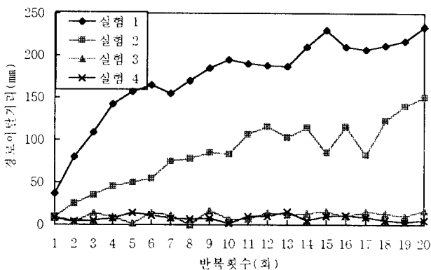
그림 5. 경로 오차 비교 Fig. 5. Comparison of navigation path errors
