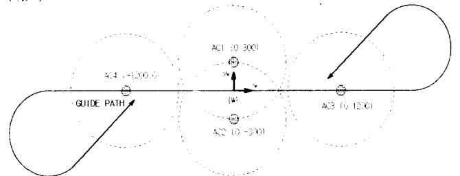
그림 4. 광원 배치 및 주행경로(단위는 mm)
