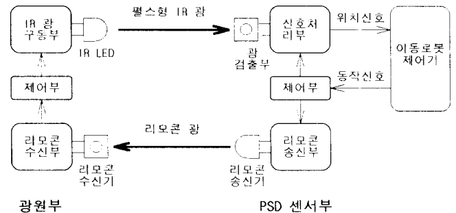
그림 1. PSD 센서 시스템 구성 Fig. 1. Structure of the PSD sensor system
