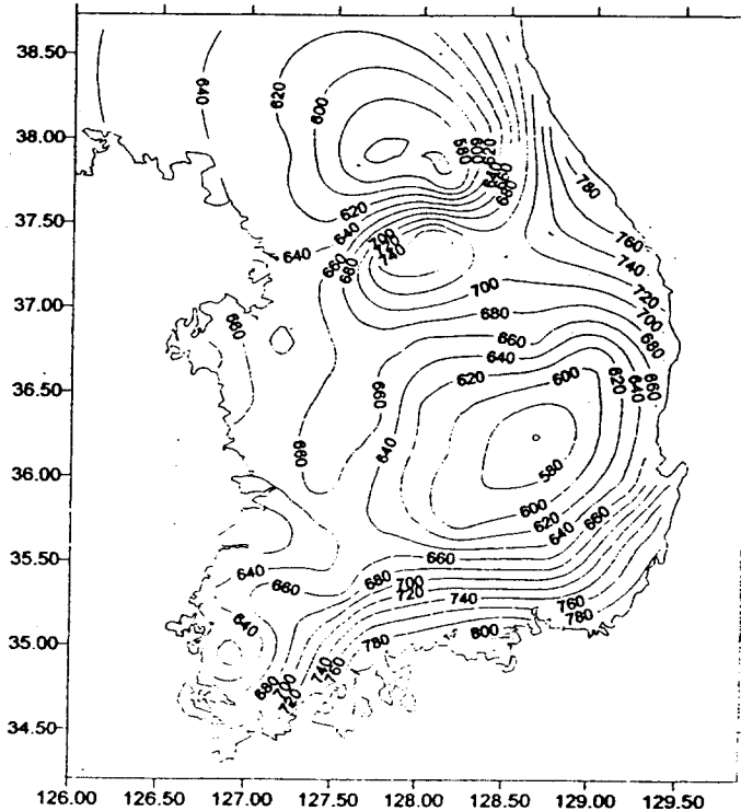
그림 2. 전국 확률 가뭄우량도
