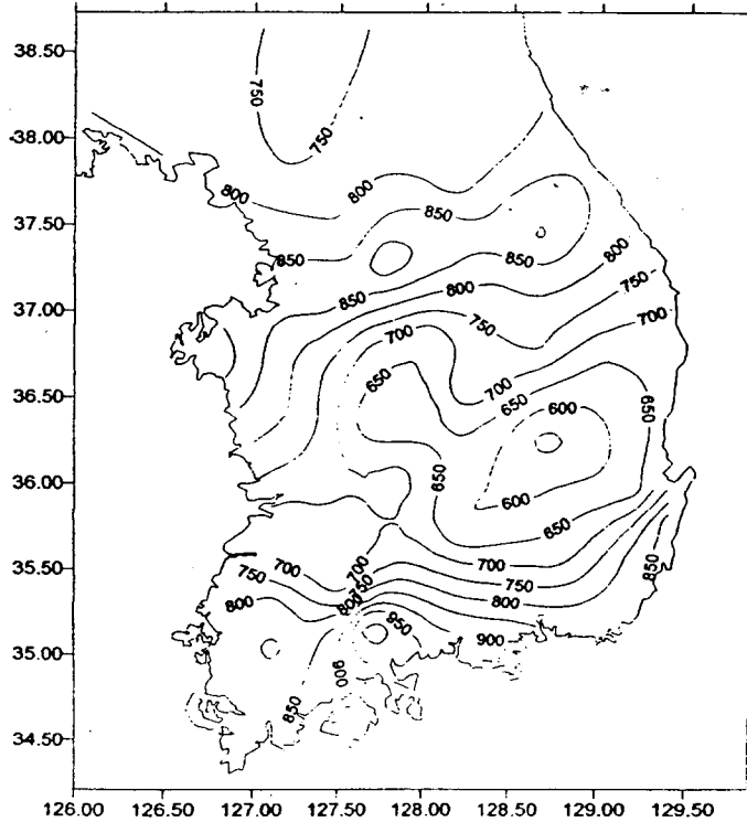
그림 3 '94-'95 가뭄기간동안의 12개월 최소 강우량
