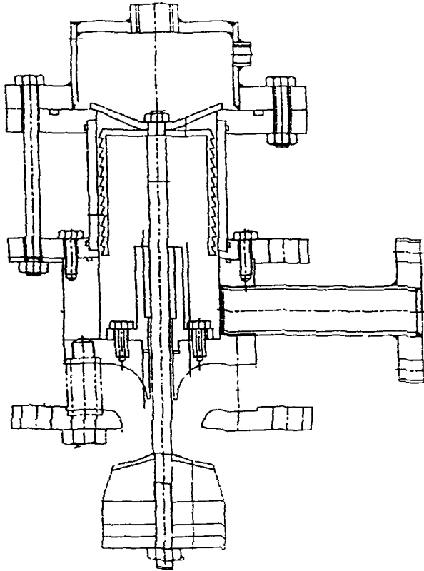
그림 1 Hydraulic Valve 전체 단면도
