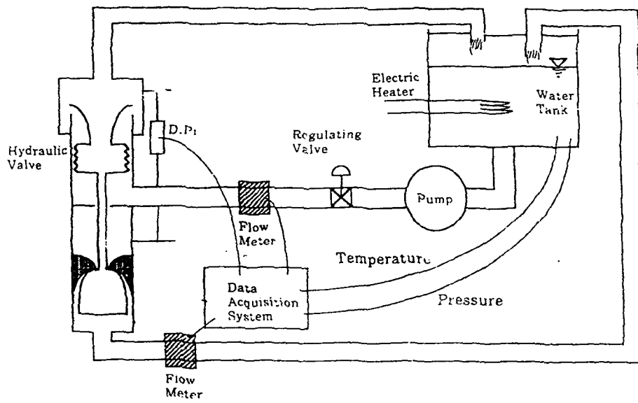
그림 2 실험장치 개략도
