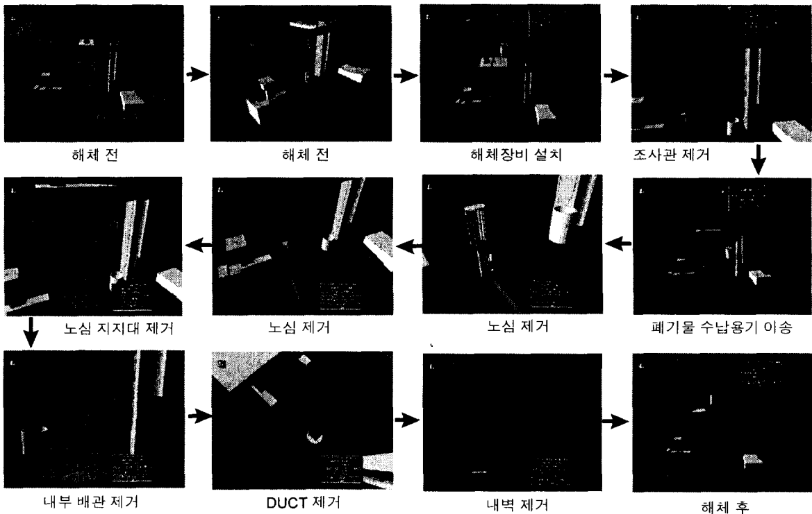
그림 6 연구로 TRIGA MARK 3 해체공정 전산모사 Fig. 6 Graphic simulation of TRIGA MARK 3 dismantling
