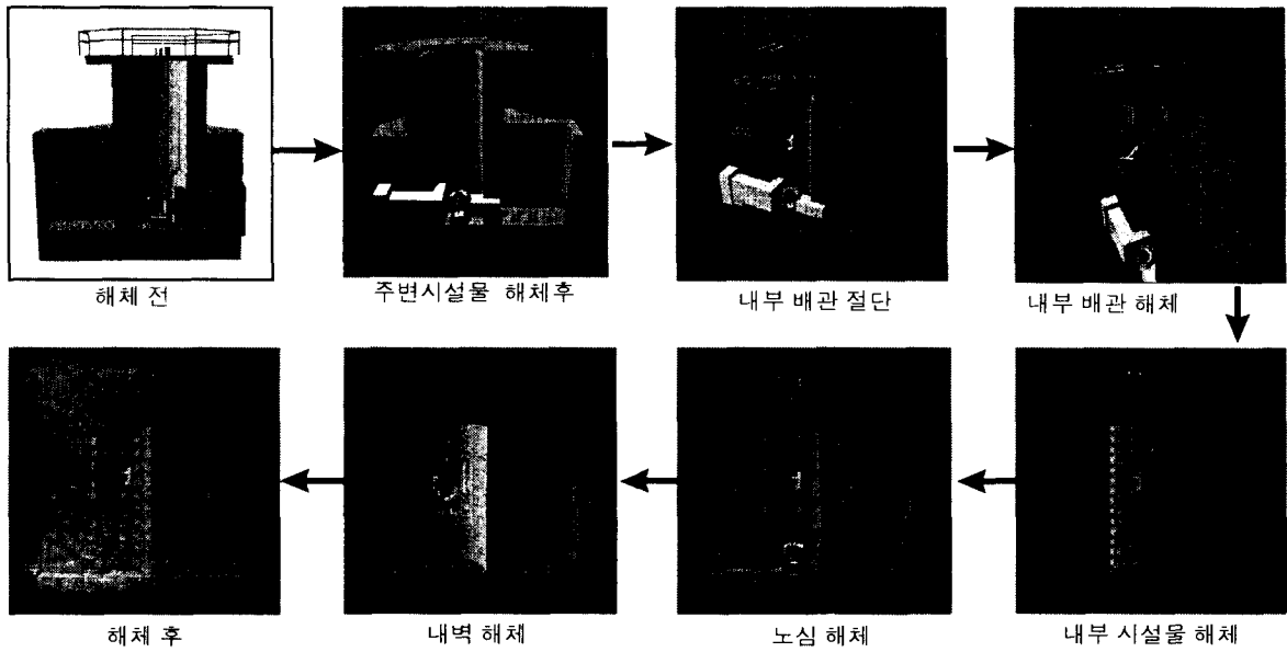
그림 5 연구로 TRIGA MARK 2 해체공정 전산모사 Fig. 5 Graphic simulation of TRIGA MARK 2 dismantling
