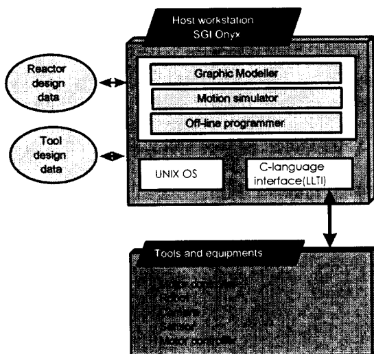
그림 1 그래픽 전산모사 시스템 구성
