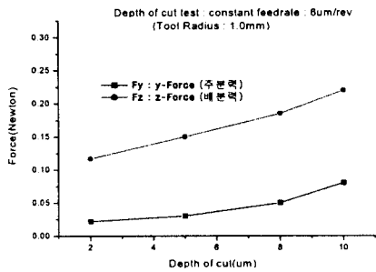
(d) Copper, Tool nose radius=1.0mm
