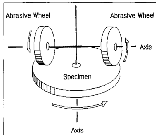
그림. 2 데이버씨 마모시험의 모식도
