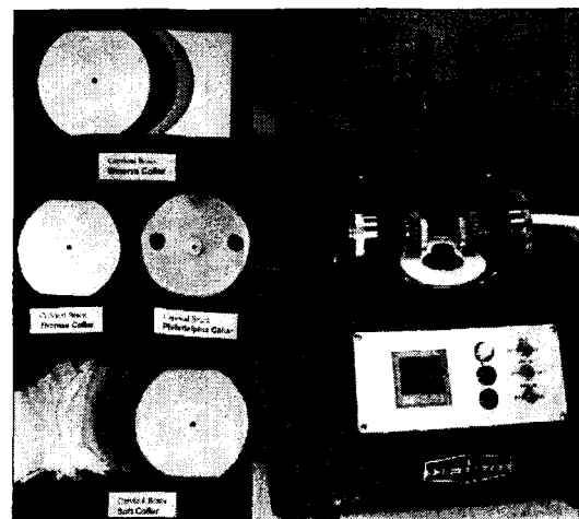
그림. 3 마모시편(A) 및 데이버씨 시험기
