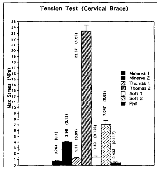
그림. 5 경추보조기의 인장강도
