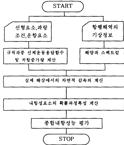
Fig. 1 기상정보에 의한 선박종합내항성능 평가 시스템의 구성
