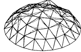
3차 모드( T_1 = 0.0953 \text{ sec} )
