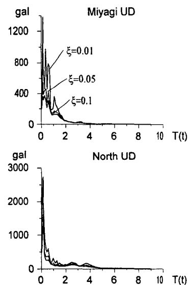
그림 7. 가속도 응답 스펙트럼
