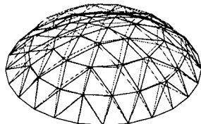
1차 모드( T_1 = 0.1054 \text{ sec} )
