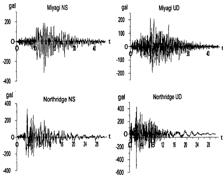
그림 6. 지진파의 가속도 시간 이력
