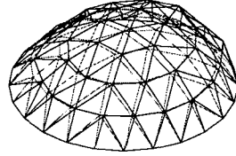
2차 모드( T_1 = 0.1053 \text{ sec} ) c) 반개각 60° 인 경우
