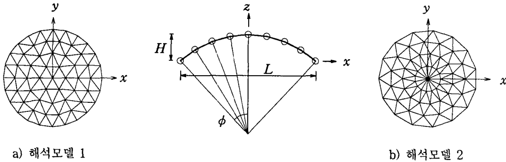
그림 2. 해석모델의 형상
