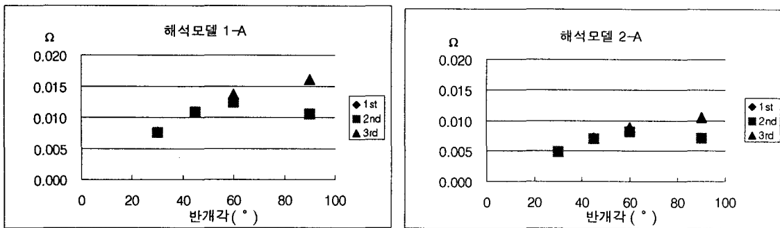
그림 5. 무차원화 진동수 \Omega 와 반개각과의 관계
