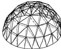
2차 모드( T_1 = 0.1229 \text{ sec} )
