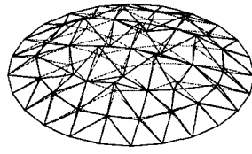
2차 모드( T_1 = 0.1727 \text{ sec} ) a) 반개각 30° 인 경우
