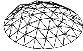
3차 모드( T_1 = 0.1195 \text{ sec} )
