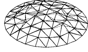
3차 모드( T_1 = 0.1694 \text{ sec} )
