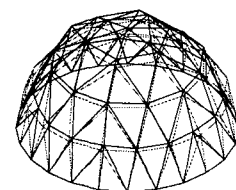
3차 모드( T_1 = 0.0811 \text{ sec} ) d) 반개각 90° 인 경우
