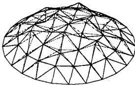
1차 모드( T_1 = 0.1198 \text{ sec} )
