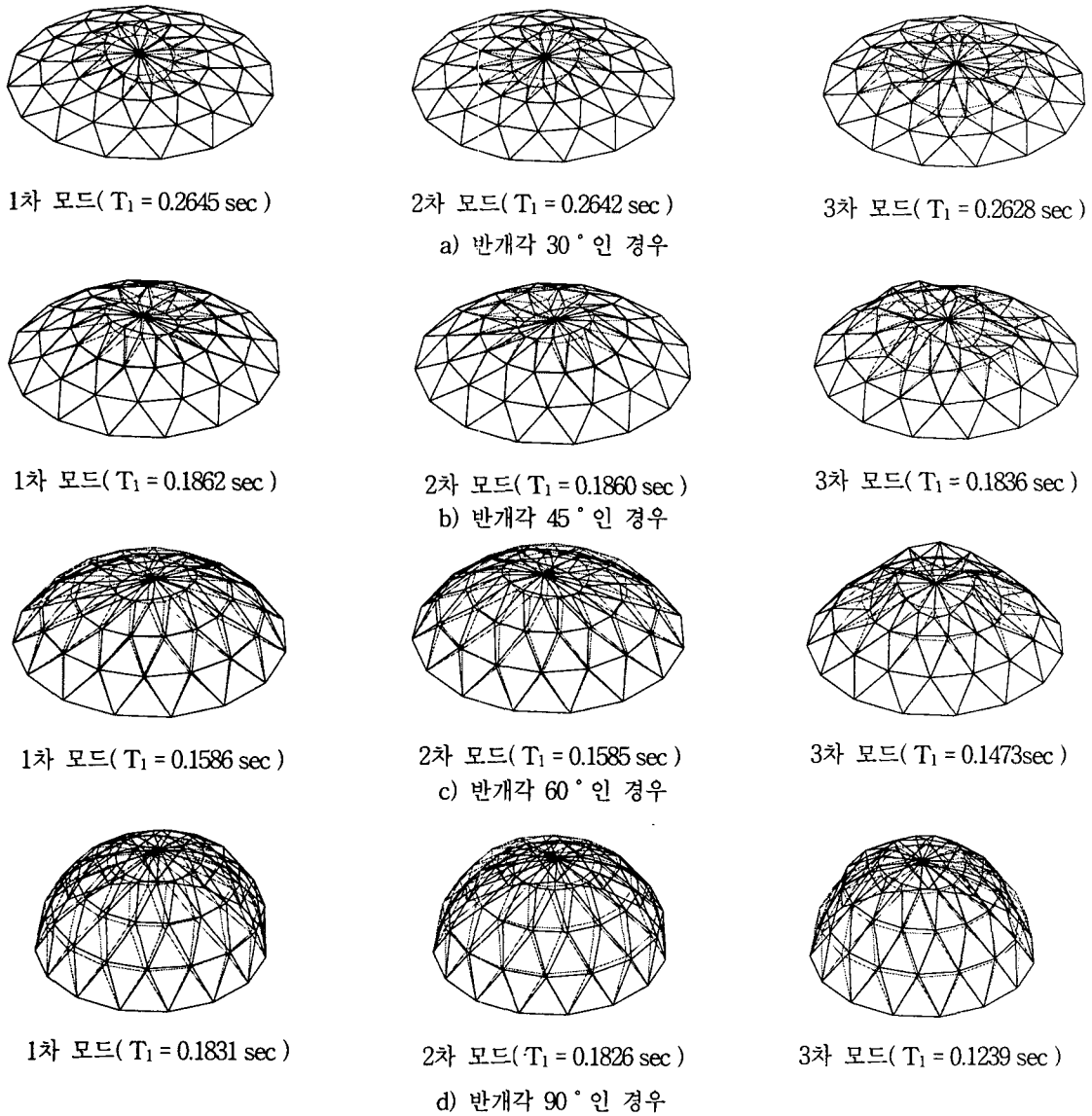
그림 4. 해석모델 2-A 의 높이/스팬비에 따른 고유모드와 고유주기
