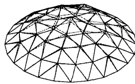
2차 모드( T_1 = 0.1196 \text{ sec} ) b) 반개각 45° 인 경우
