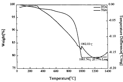
그림 3. SrTiO 3 분말의 시차열분석 및 열중량분석
