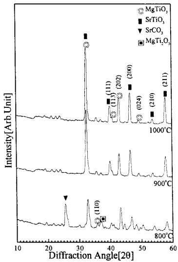
그림 4. 하소온도를 변화시킨 0.8MgTiO 3 -0.2SrTiO 3 분말의 X-선 회절모양
