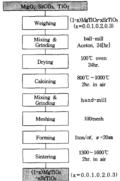
그림1. MgTiO 3 -SrTiO 3 세라믹의 제조과정
