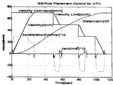
그림 6. GS-극배치기법에 의한 속도추종
