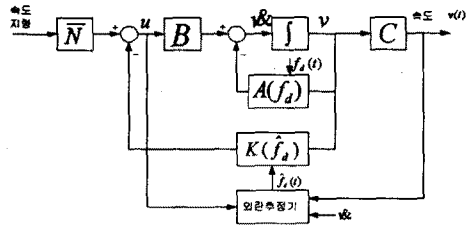
그림 4. GS-극배치 제어기
