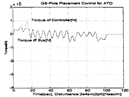
그림 10. 외란적용시 GS-PP 요구토크
