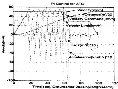
그림 7. 외란적용시 PI제어특성
