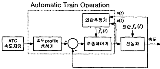
그림 2. 열차제어 구성도
