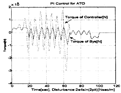
그림 9. 외란적용시 PI제어 요구토크
