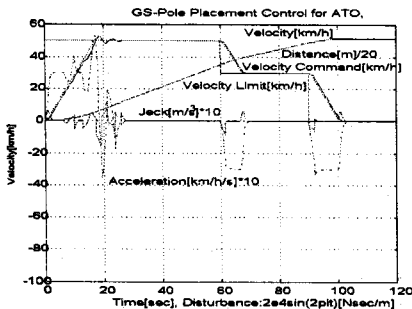
그림 8. 외란적용시 GS-PP 제어특성
