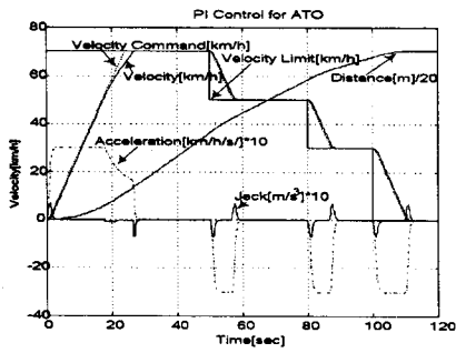
그림 5. PI제어에 의한 속도추종
