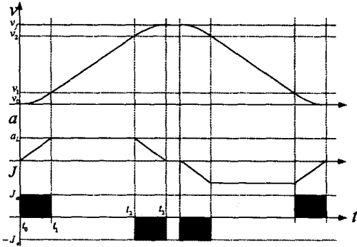
그림 3. 속도 profile
