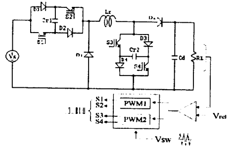
그림 3 소프트 스위칭에 의한 승·강압 초퍼회로 Fig. 3 The buck·boost chopper circuit by soft-switching
