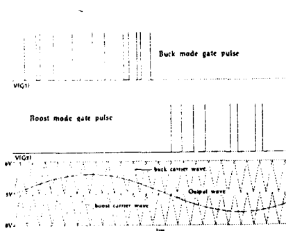
그림 6 승·강압 PWM제어동작파형 Fig 6 The operating wave form of buck-boost PWM control
