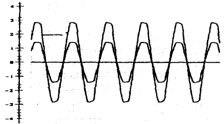
그림 18 인버터 출력전압, 전류 Fig. 18 output voltage and current of inverter
