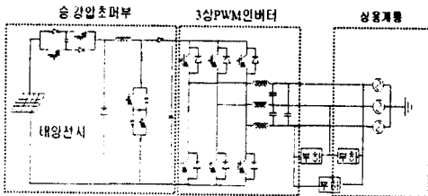
그림 1. 부분공진기법을 이용한 트랜스리스 계동연계 인버터의 회로
