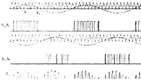
그림 14 인버터부의 제어신호와 전류파형 Fig. 14 Control signals and current waveform of Part of inverter
