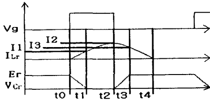
그림 4 부분공진 승·강압 초퍼의 이상적인 파형
