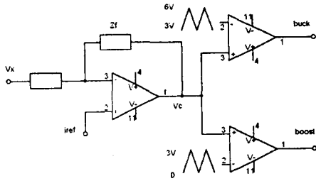
그림 5 제어부의 OP-AMP구성 Fig. 5 The OP-AMP configuration of a part of control
