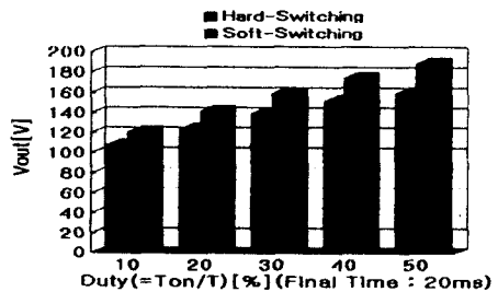
그림 13 듀티율변화에 따른 출력전압 비교 Fig. 13 The comparison for output voltage according to changing duty ratio
