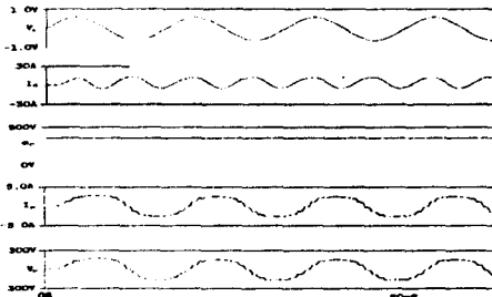
그림 15 입.출력 전압, 전류파형 Fig. 15 Simulation Waveforms of voltage and current
