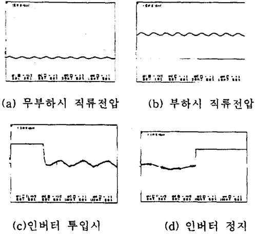
그림 16 계통연계시 특성 Fig. 16 Characteristics of The Utility Interactive
