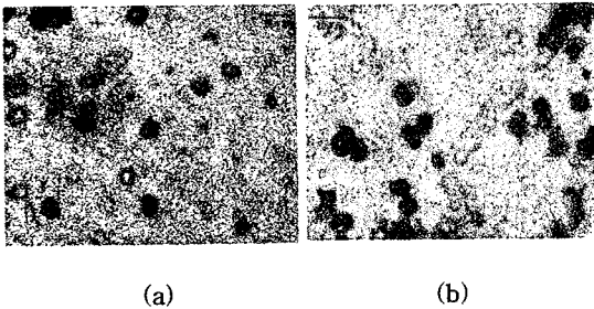
그림 3. (a)수직브리지만법에 의해 성장된 InSe결정 (b)InSe:Sn (110) 면에 나타난 에치피트 (×400) Fig 3. (a)InSe crystal grown by vertical Bridgman method (b)Etch pits revealed on (110) InSe:Sn surface (×400)
