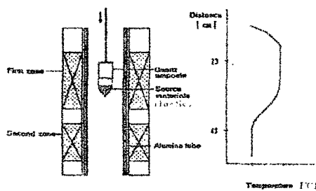
그림 1. InSe 결정성장용 수직 브리지만 전기로와 온도구배의 개략도
