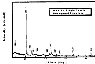
그림 4. InSe:Sn 결정의 X-선 회절 패턴
