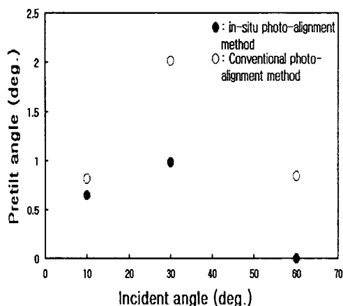
그림 2. 폴리이미드 표면에 UV광 조사에 따른 네마틱 액정의 프리틸트각의 조사각도 의존성 Fig. 2. Dependence of incident angle of NLC pretilt by UV light irradiation on PI surfaces.
