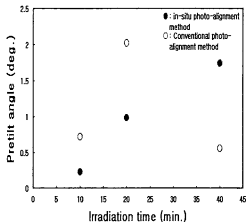
그림 3. 폴리이미드 표면에 UV광 조사에 따른 네마틱 액정의 프리틸트각의 조사시간 의존성 Fig. 3. Dependence of irradiation time of NLC pretilt by UV light irradiation on PI surfaces.
