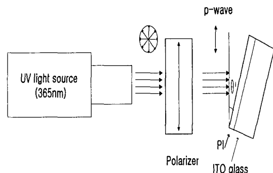
그림 1. UV 광조사 시스템.
