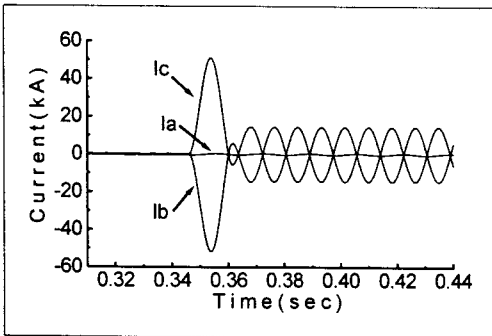
그림 2. 저항형 초전도 한류기를 적용한 선간 단락사고 (사고각 0^\circ )
