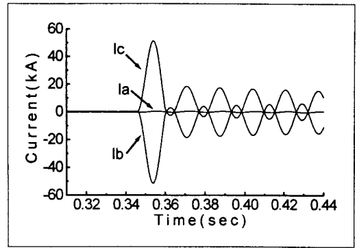
그림 3. 유도형 초전도 한류기를 적용한 선간 단락사고 (사고각 0^\circ )
