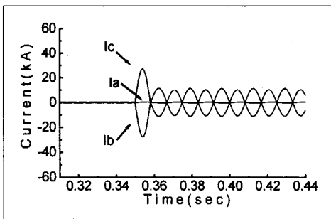
그림 7. 유도형 초전도 한류기를 적용한 선간 단락사고 (사고각 90°)
