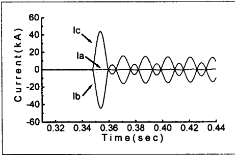
그림 5. 유도형 초전도 한류기를 적용한 선간 단락사고 (사고각 45°)
