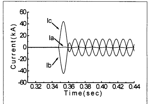
그림 4. 저항형 초전도 한류기를 적용한 선간 단락사고 (사고각 45^\circ )
