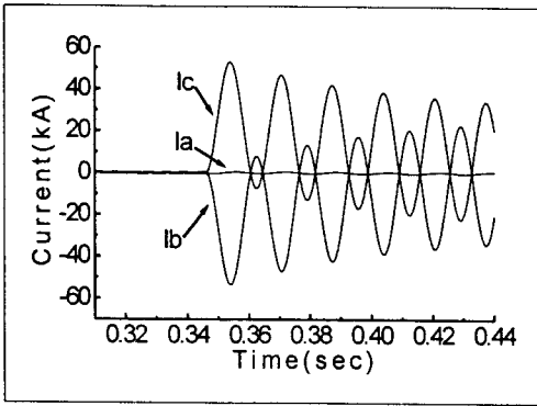
그림 1. 사고각 0^\circ 일때의 고장전류 파형
