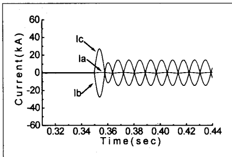
그림 6. 저항형 초전도 한류기를 적용한 선간 단락사고 (사고각 90°)
