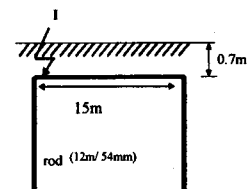
(c) XIT 접지(습식전해질) 구조
