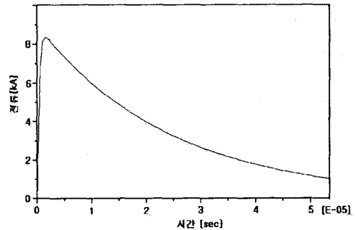
그림 2.10 임펄스 전류 파형 Fig. 2.10 Impulse Current Wave
