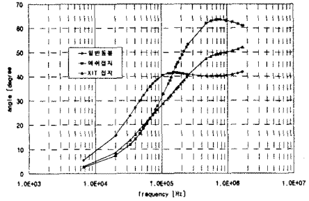
(b) 접지임피던스 위상 응답
