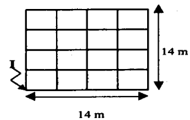
(b) 메쉬접지 구조
