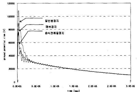
그림 2.11 유입점에서의 접지극 전위상승 Fig. 2.11 Ground Potential Rise
