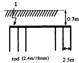
(a) 일반동봉접지 구조
