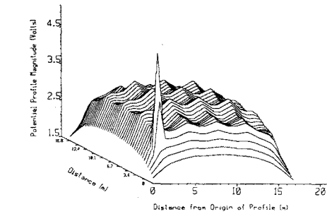
그림 2.6 지표면 전위상승 60Hz (메쉬접지) Fig. 2.6 Earth surface potential at 60 Hz (Mesh)
