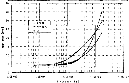
(a) 접지임피던스 크기
