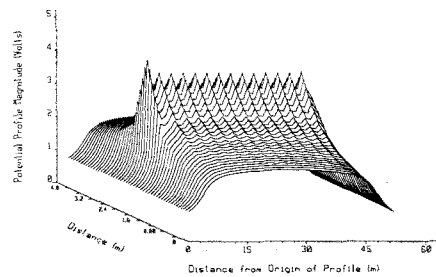
그림 2.4 지표면 전위상승 60Hz(일반동봉) Fig. 2.4 Earth surface potential at 60 Hz (rod systems)
