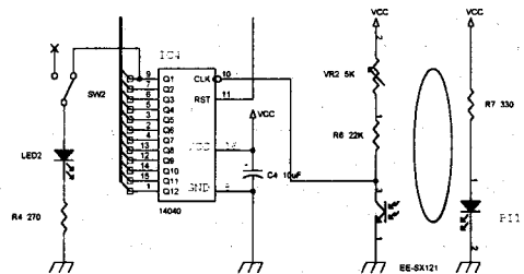
그림 5. 12BIT COUNTER CIRCUIT
