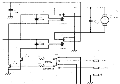
그림 6. DC MOTOR DRIVER CIRCUIT
