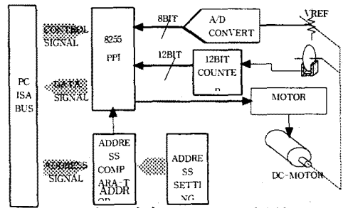
그림 1. 전체 BLOCK DIAGRAM
