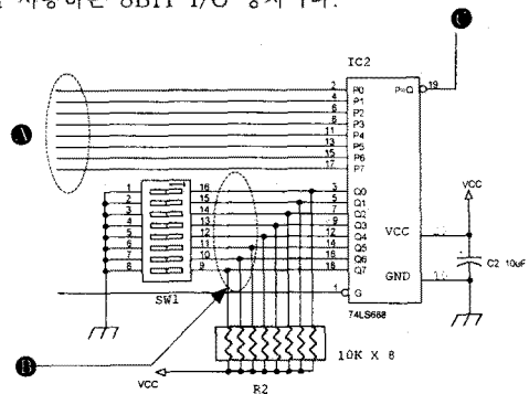
그림 2. ADDRESS COMPARATOR CIRCUIT
