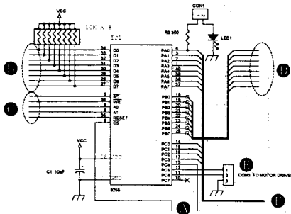
그림 3. I/O INTERFACE CIRCUIT
