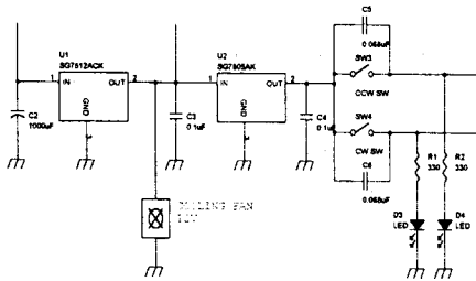
그림 7. DC MOTOR DRIVER CIRCUIT
