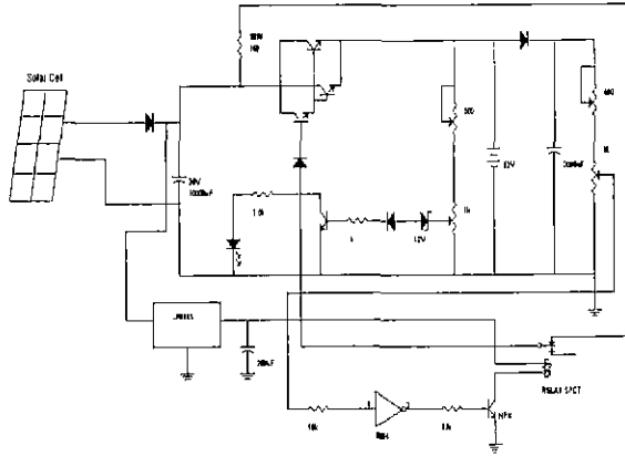
그림 6 태양전지 충전회로의 구성도 Fig. 6 Circuit of Charge with PV Module
