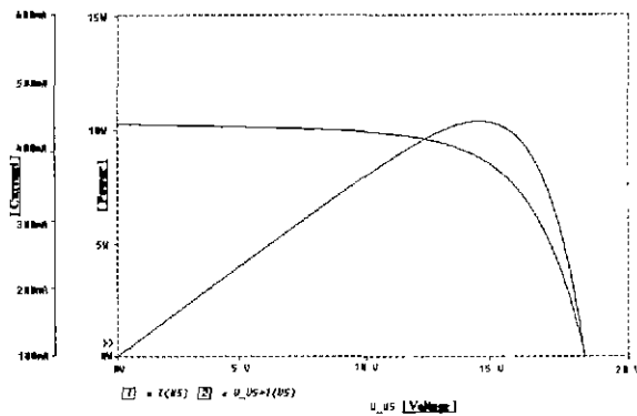
그림 7 태양전지의 V-I 특성곡선 및 전력곡선 Fig. 7 Curve of V-I Characteristic and Power with PV Module
