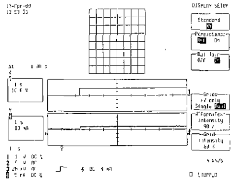
그림 8 PV Module의 V-I 실험파형 Fig. 8 Experiment form of V-I with PV Module
