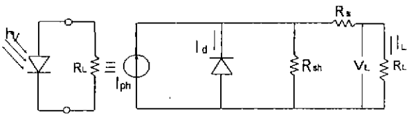
그림 2 태양전지의 등가회로 Fig. 2 Equivalent Circuit of Solar Cell
