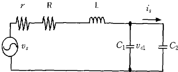
그림 2 부하등가회로
