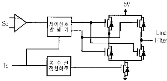
그림 3 광대역통신용 새로운 증폭기의 블록선도
