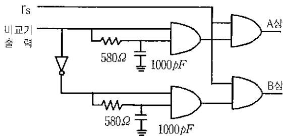
그림 4 제어신호 발생기
