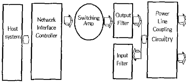
그림 1 PLC 시스템 블록선도
