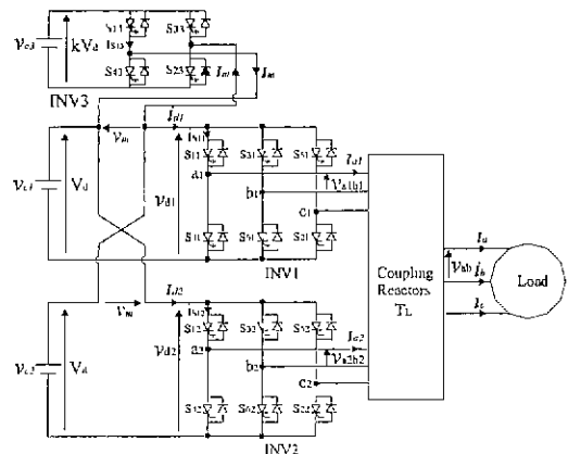
그림 1 제안한 36-스텝 인버터 Fig 1. Proposed 36-step Inverter
