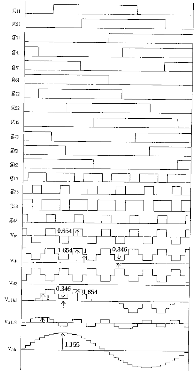
그림 2. 제안한 36-스텝 인버터의 주요파형 ( V_d=1 , I_a=1 , k=0.654 일 때)
