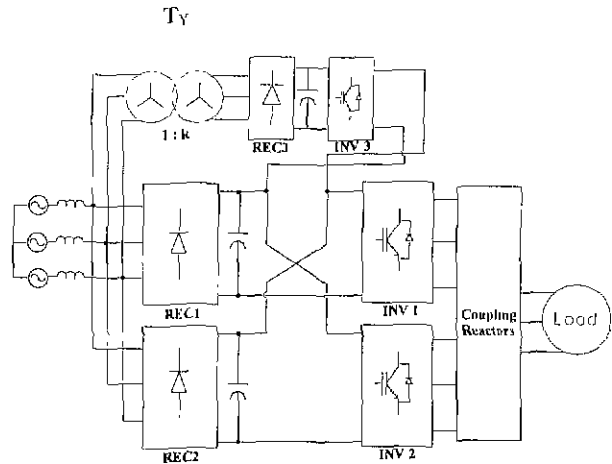
그림 5 제안하는 정류기-인버터 시스템
