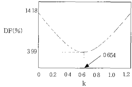
그림 4. 보조회로의 전압비 k 에 따른 출력전압의 왜곡률
