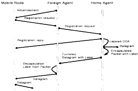
[그림 4] MPLS기법을 사용한 이동 IP에서의 Data 전송
