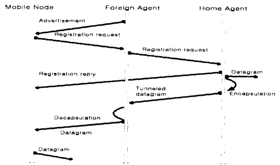
[그림 3] 이동 IP에서의 Data전송
