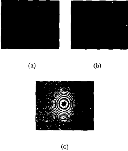
그림 5 실험에 의해 변형 삼각간섭계에서 얻어진 간섭 패턴 (a) \Gamma_1 = 0 , \Gamma_2 = \frac{\pi}{2} 인 경우의 점광원 홀로그램 (b) \Gamma_1 = 0 , \Gamma_2 = -\frac{\pi}{2} 인 경우의 점광원 홀로그램 (c) (b)에서 (a)를 뺀 영상.
