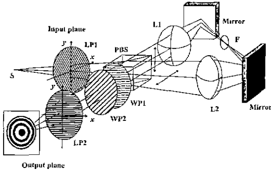
그림 1. 변형 삼각 간섭계
