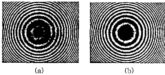
그림 3. 변형 삼각 간섭계로부터 얻은 복소홀로그램 (a) 실수부 (b) 허수부
