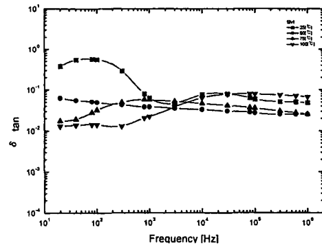
그림 5. 유전정접의 주파수 의존성 (접합시료, 5[V])
