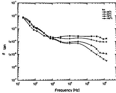
그림 3. 유전정접의 주파수 의존성 (XLPE, 5[V])
