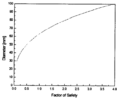
그림 3. 안전율에 따른 FRP 봉의 직경
