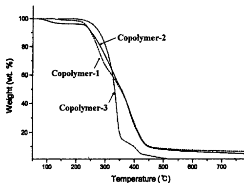
그림 2 3종류의 공중합체의 TGA 특성.
