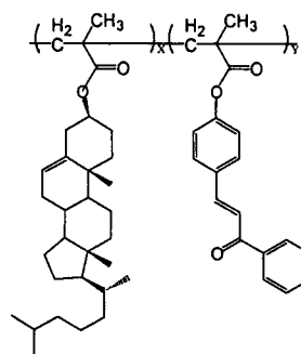
그림 1 공중합체의 분자구조.
