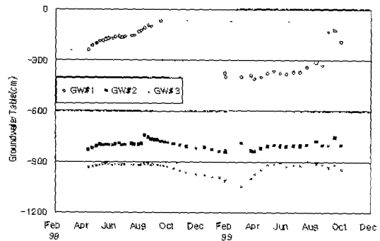
그림 9. 시험지구 지하수위 변화
