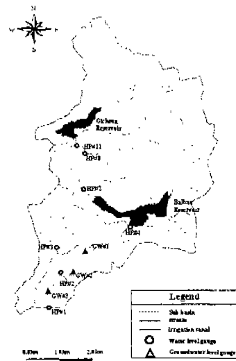
그림 2. 시험지구 수문계측망
