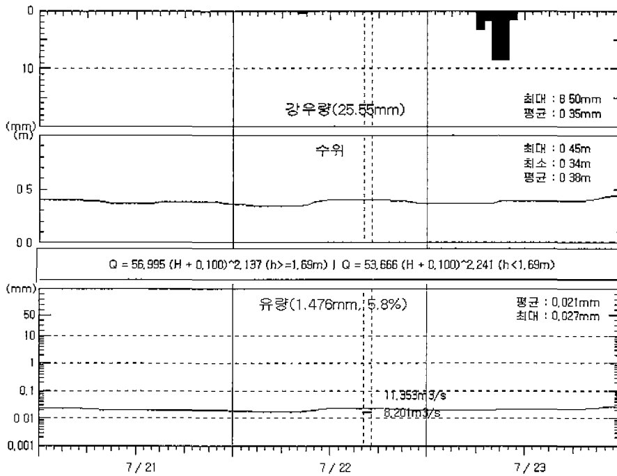
그림 2 수문곡선 중첩예(호탄, 1999.7.22)
