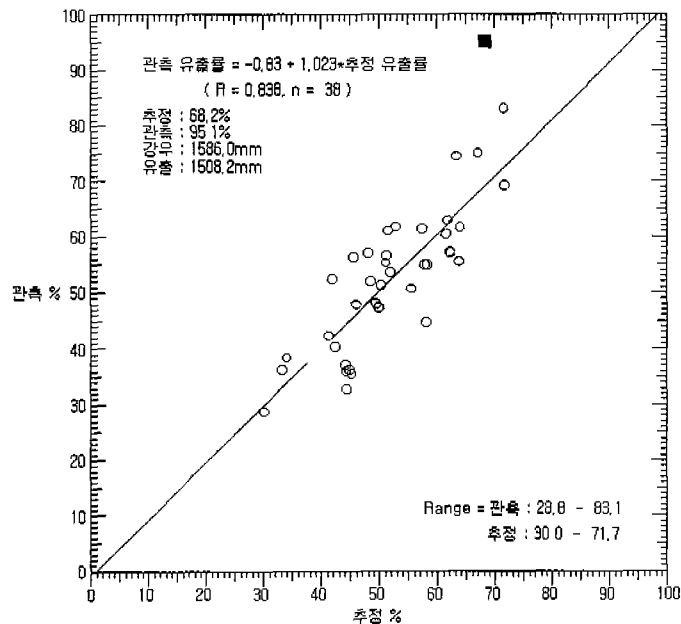
그림 8 유출률 공식(금강)에 의한 평가 예(1998, 옥천)
