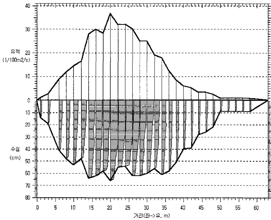
그림 1 유량 계산 예(호탄, 1999.7.22)
