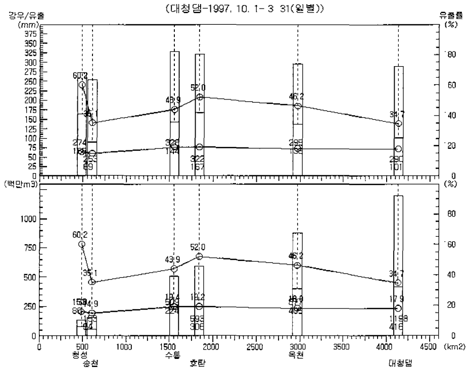
그림 4 댐 유역내 유출량 비교(대청댐, 1997.10.1-31)
