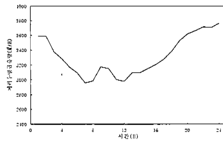
[그림 6] 시간별 하수처리량의 변화(천안, 1999)
