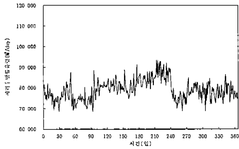
[그림 3] 일별하수처리량의 변화(천안,1998)
