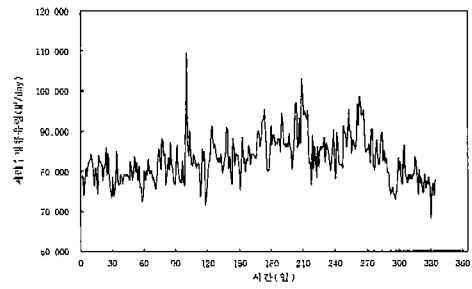
[그림 4] 일별하수처리량의 변화(천안, 1999)
