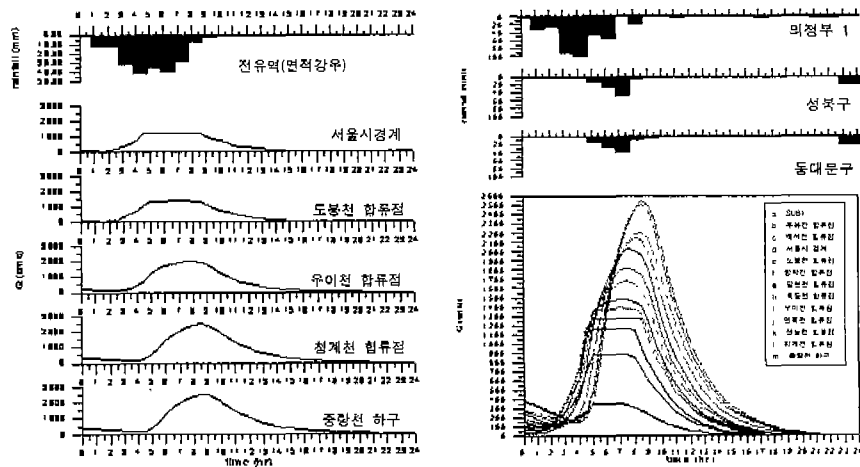
그림 2 '98년 8월 6일 유출수문곡선(중랑천)
