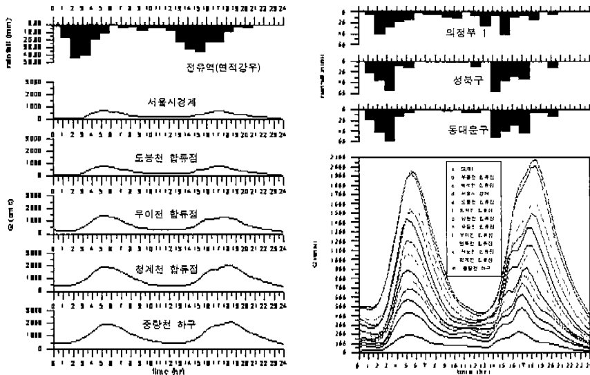
그림 3 '98년 8월 8일 유출수문곡선(중랑천)
