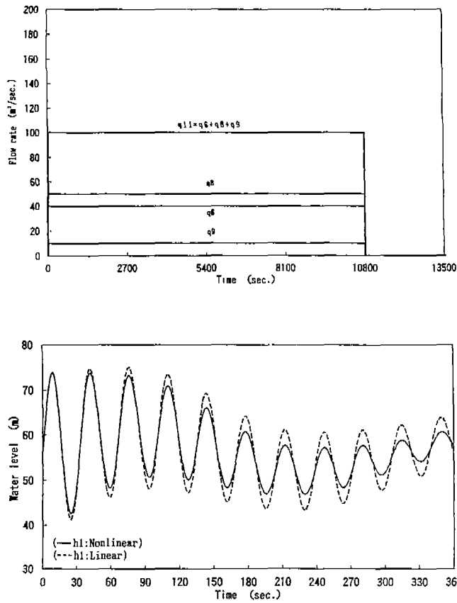
그림 2 비선형계와 선형계의 비교(장방형 펄스상의 유입, 유출에 의한 해석)
