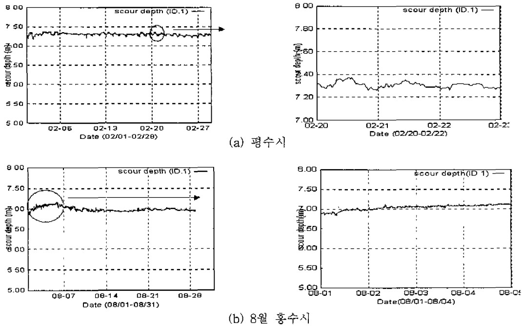
그림 3 한남대교 구간의 세굴량 자료
