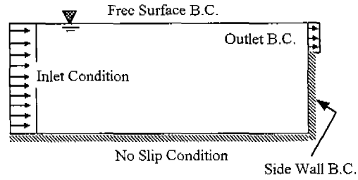
그림2. SS모델해석을 위한 침전지 도식도
