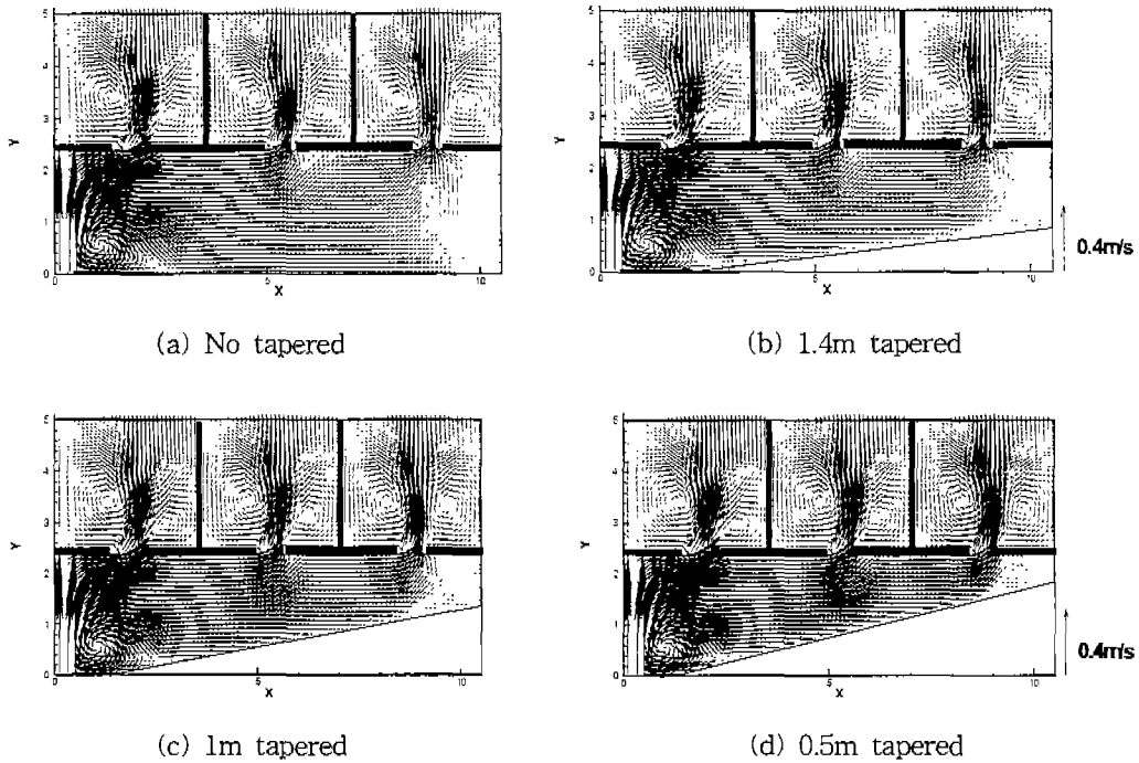
그림6. Vector plots of channel
