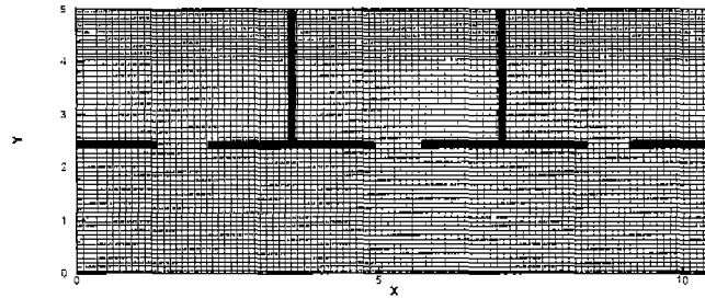
그림3. 계산영역의 mesh generating
