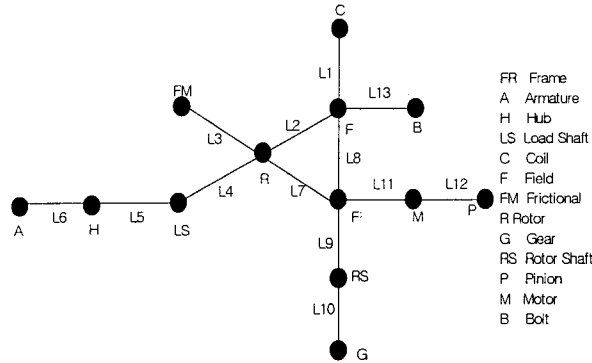
[그림 4] 전자 클러치의 리에이중 다이어그램
