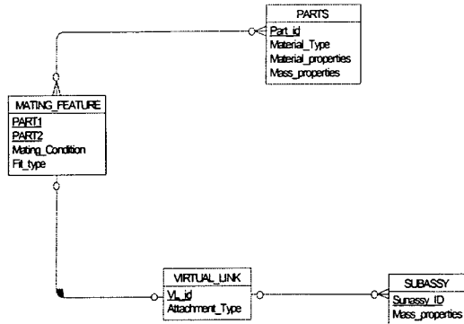
[그림 6] 가상 고리 데이터 구조
