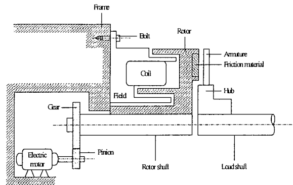
[그림 2] 전자 클러치
