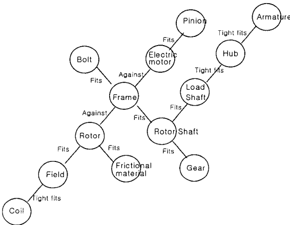
[그림 5] 전자 클러치의 선행 그래프
