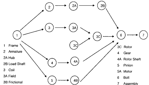
[그림 3] 전자 클러치의 선행다이어그램
