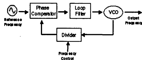
그림 1 PLL 신세사이저의 구성
