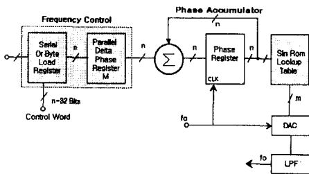
그림 3 DDS의 구성
