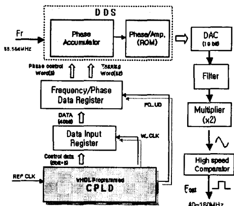
그림 4 설계된 고속 클럭 발생기의 구성
