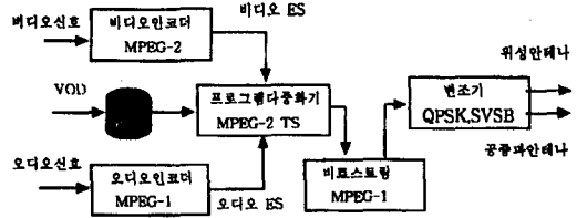
그림7. DTV 신호 전송 구성도
