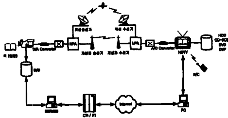
그림9. 대화형 독서출판 TV 방송 구성도
