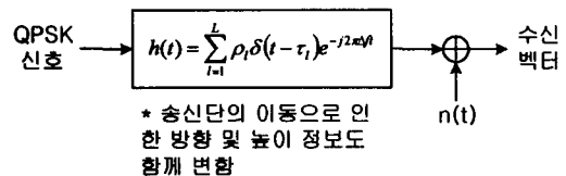
그림 6 수중 초음파 전달 모델
