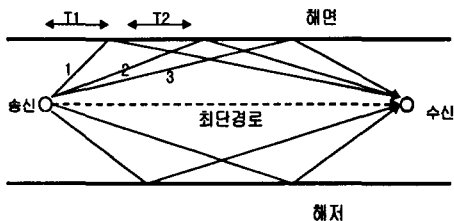
그림 5 다중경로
