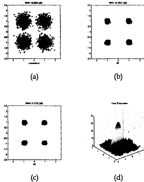
그림 9 채널 시뮬레이터 출력
