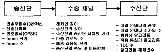
그림 1 채널 시뮬레이터 구조
