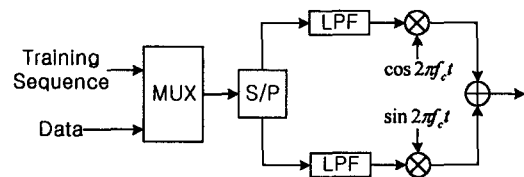
그림 2 QPSK 변조기의 구조
