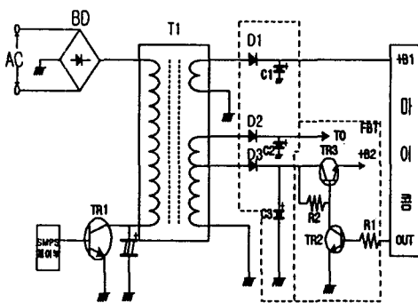
그림2. TV에서의 기존의 대기전력 차단 회로
