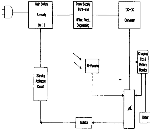
그림3. 대기전력 차단회로의 개략도
