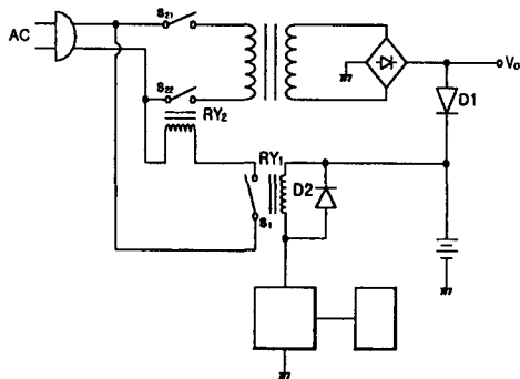
그림4. 대기전력 차단회로도
