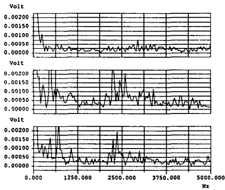
그림 3. 전대역 주파수 변화(상:배경잡음, 중:삽입전, 하:삽입후)
