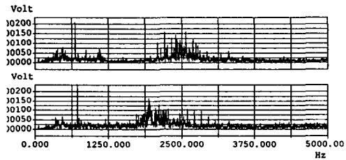
그림 5. 철판 삽입전,후 주파수대역내 분포 변화 Fig. 6 Fluctuations of frequency using a piece of iron
