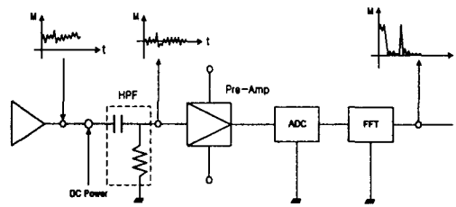
그림2. 이물질 감지시스템 동작구성도
