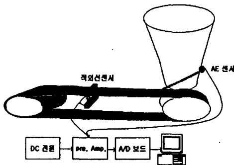
그림 1. 감시 시스템 개략도
