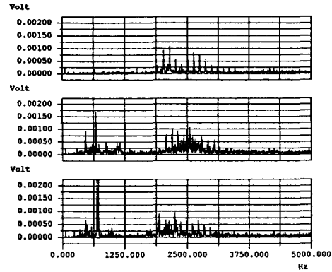
그림 4. HPF를 이용한 후 전대역 주파수 변화 Fig. 4 Fluctuations of frequency after using HPF
