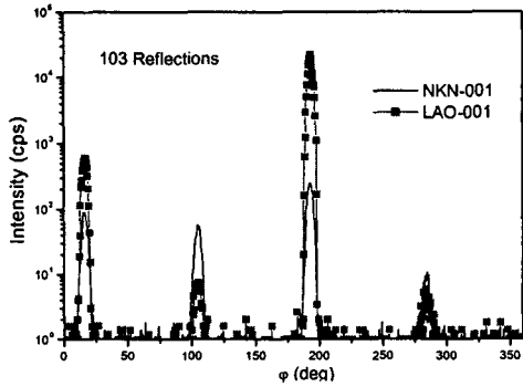
그림 4. NKN-(103)면에 대한 \phi -scan X-선 회절 모양.
