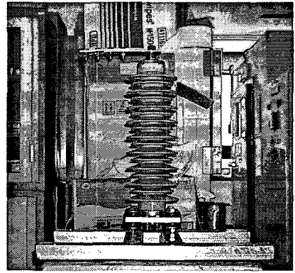
그림 3. 개발된 전철용 피뢰기의 외관
