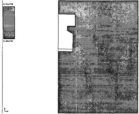
그림 2. 피뢰기의 전계분포
