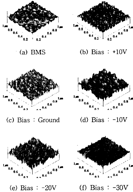
그림 8. 기판 bias 전압에 따른 MgO 표면 AFM 사진
