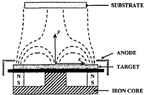
그림 2. 불평형 마그네트론 스파터링의 개략도
