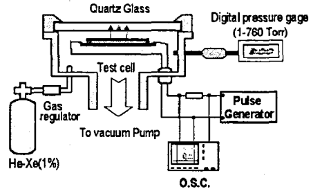
그림 4. 방전 챔버의 개략도
