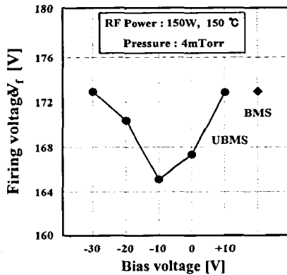
그림 6. 기판 Bias 전압에 따른 방전개시 전압
