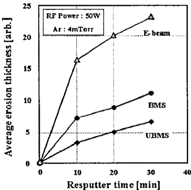
그림 9. MgO 제작 방법에 따른 내스파터링 특성
