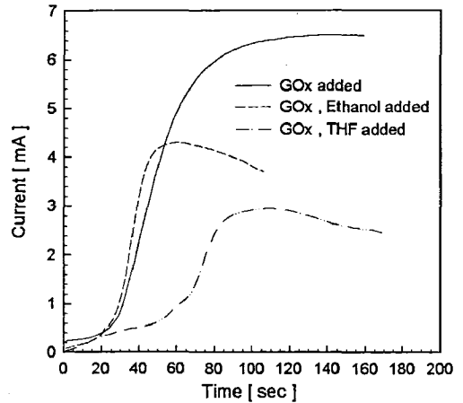
그림 2. PPy-GOx 효소전극의 전해중합 동안 전류의 경시적 변화. Fig. 2. Chronoamperometry for PPy-GOx enzyme electrode. film growth.
