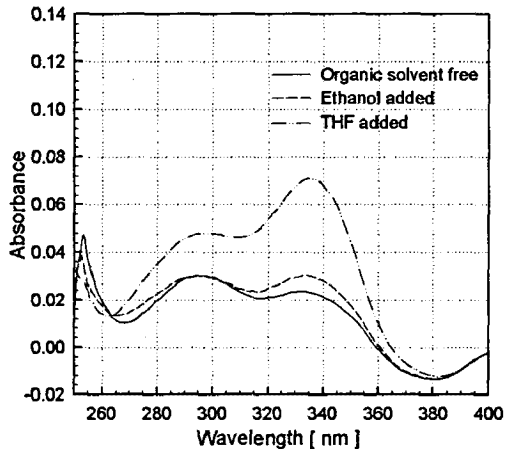
그림 5. 중합 후 pyrrole oligomer에 대한 자외선 흡수 스펙트럼. Fig. 5. UV absorption spectra of pyrrole oligomer in the solution after synthesis.
