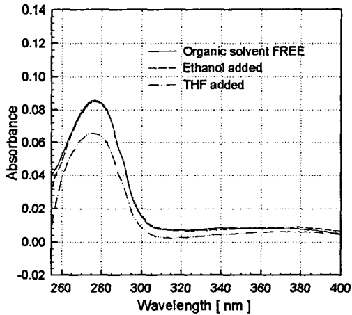
그림 3. 중합액의 중합 전 자외선 흡수 스펙트럼. Fig. 3. UV absorption spectra of the synthetic solution before synthesis.
