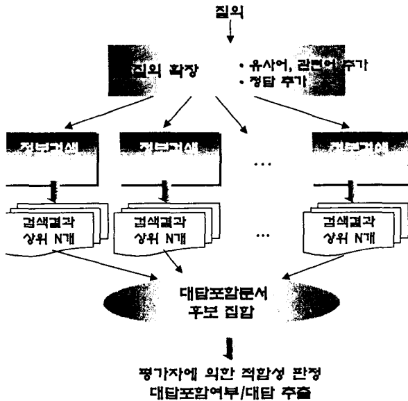
그림 1. 문서검색결과 조합방법을 이용한 답포함문서 후보집합 생성 과정
