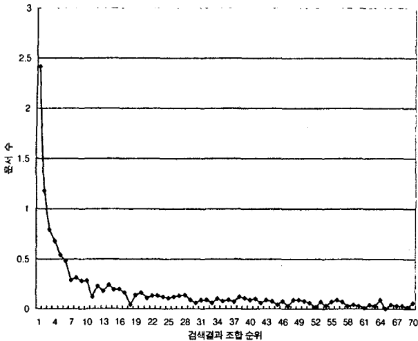
그림 4. 상위문서 수의 변화에 따라 평균적으로 추가되는 대담포함문서 개수
