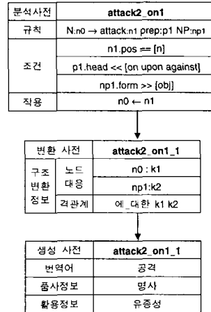
그림 5: 복합 관용어구 규칙의 예제
