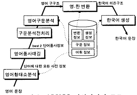
그림 2: ALKOL 번역서버의 구조
