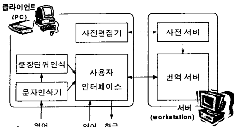
그림 1: ALKOL의 시스템 구조
