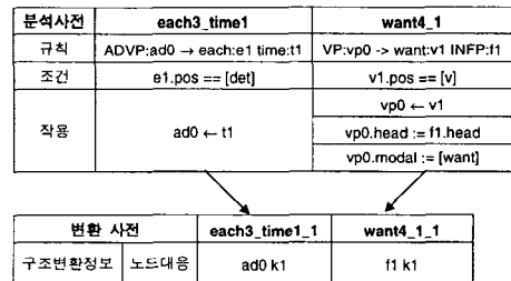
그림 6: 단순 관용어구와 양상 자질 관련 규칙 예제
