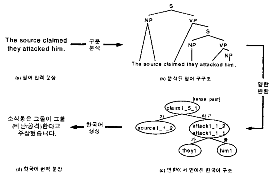
그림 8: ALKOL의 번역 예제
