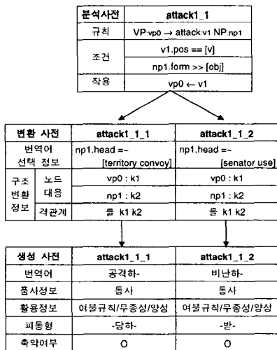
그림 4: 단순 동사구 규칙의 예제
