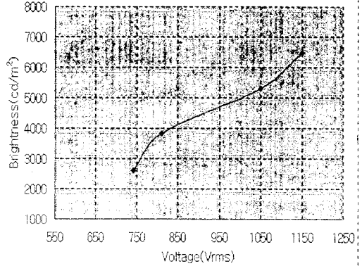
그림 4 전압에 따른 휘도 특성
