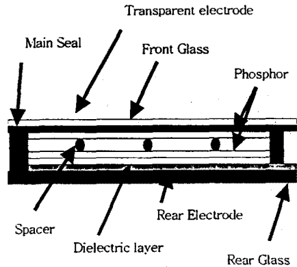
그림 1 램프의 구조 Fig. 1 construction of Lamp
