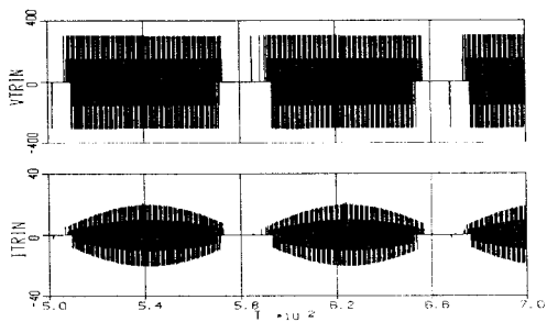
그림 4 고주파변압기의 1차측 입력전압(V trin ), 전류(I trin )
