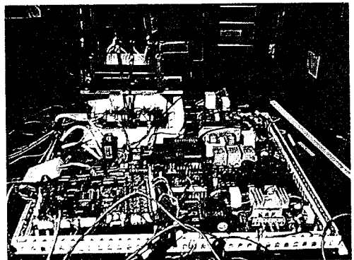
그림 8 고주파링크방식의 연계형 인버터 시제품
