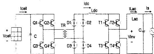
그림 2 고주파링크 방식의 연계형 인버터 토폴로지
