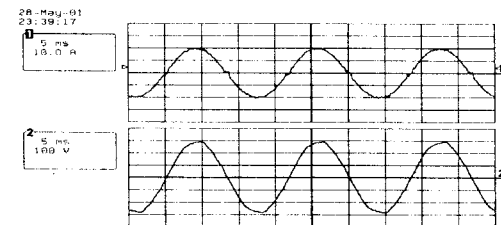
그림 13 계통전압( V_s )과 유입전류( I_s )
