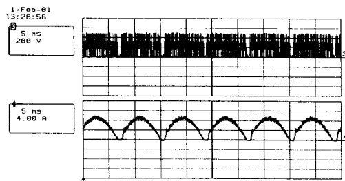
그림 11 고주파변압기의 1차측 입력전압( V_{trin} ), 전류( I_{trin} )
