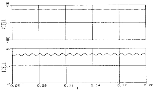
그림 3 태양전지 어레이의 전압(V cell ), 전류(I cell ) 파형
