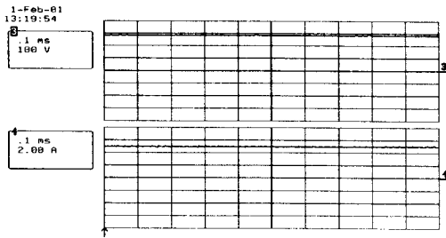
그림 9 태양전지 어레이의 전압( V_{cell} ), 전류( I_{cell} ) 파형
