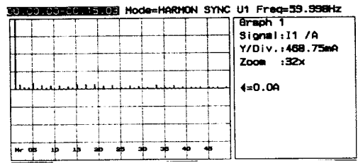
그림 14 계통 유입전류( I_s )의 THD 분포도
