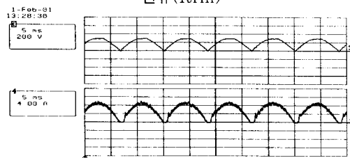
그림 12 dc리액터의 출력전압( V_{inv} ), 전류( I_{dc} )
