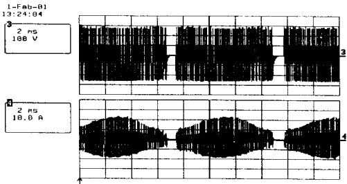
그림 10 고주파변압기의 1차측 입력전압( V_{trin} ), 전류( I_{trin} )
